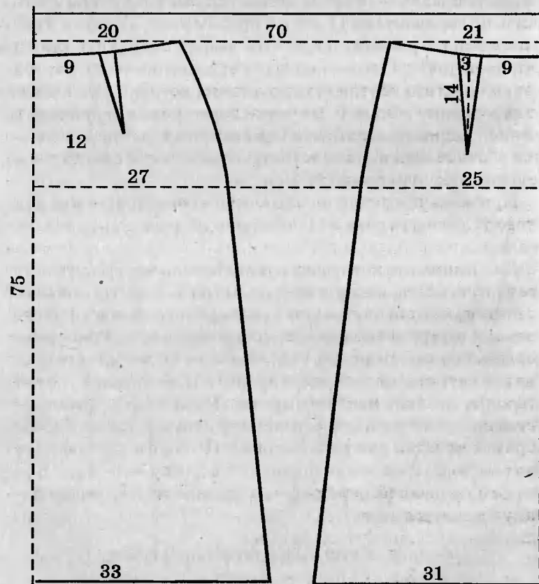
Рис. 14. Основная выкройка двучастной юбки
