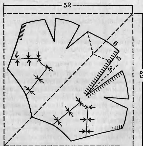
Рис. 34. Разработанный чертеж выкройки переда лифа свадебного платья
