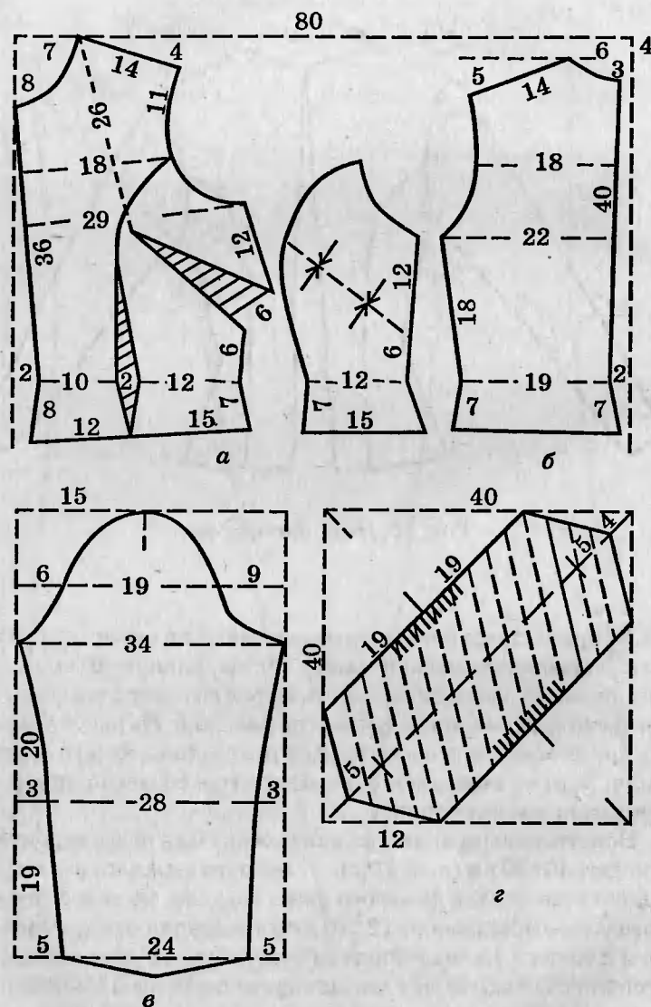
Рис. 26. Чертеж выкройки накидки фигаро
