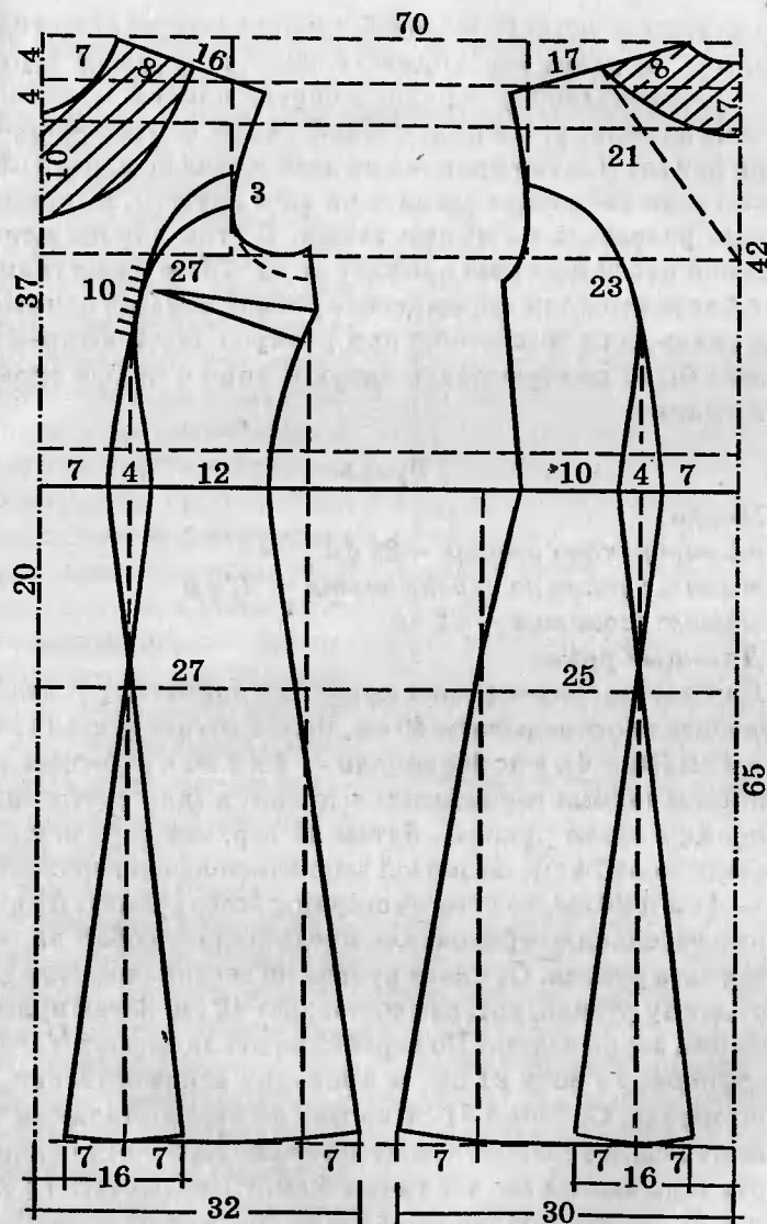
Рис. 40. Чертеж выкройки платья «принцесса»
