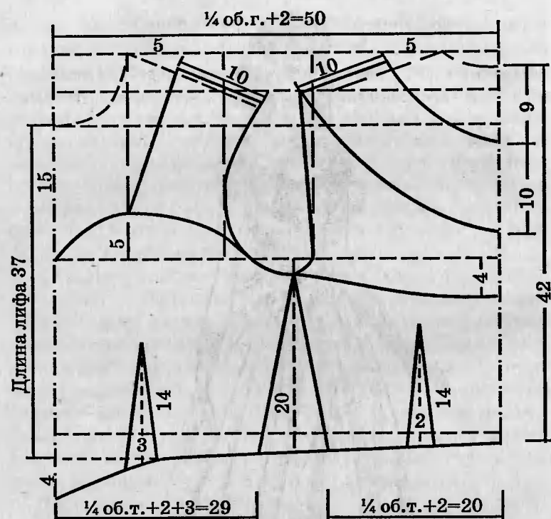
Рис. 31. Чертеж выкройки лифа свадебного платья
