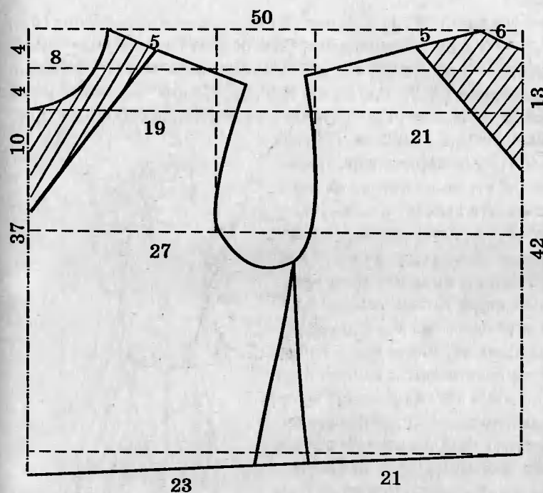
Рис. 17. Чертеж выкройки блузки с V-образным вырезом
