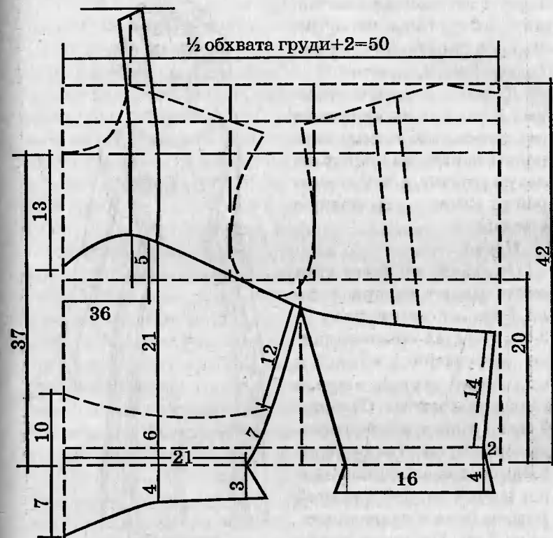
Рис. 38. Чертеж выкройки верхней части свадебного платья
