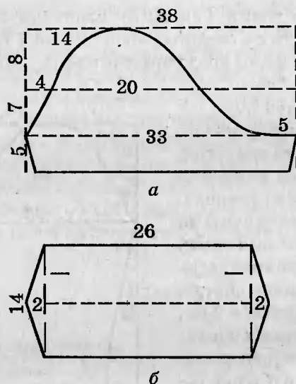
Рис. 42. Чертеж выкройки короткого рукава и манжета
